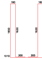
④ 1φ12 L=8510
